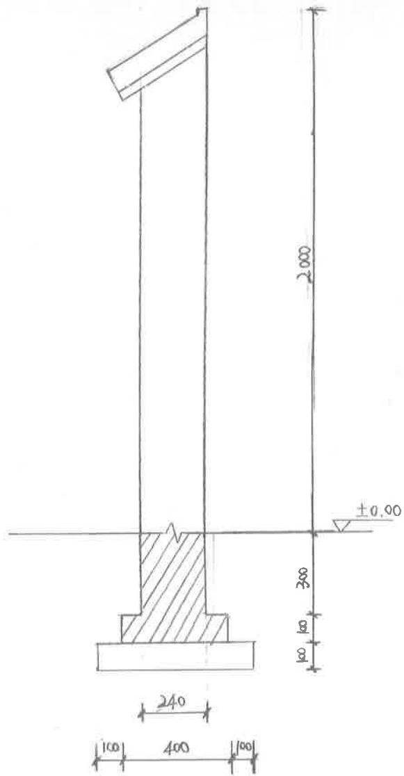
围墙剖面 1:20
