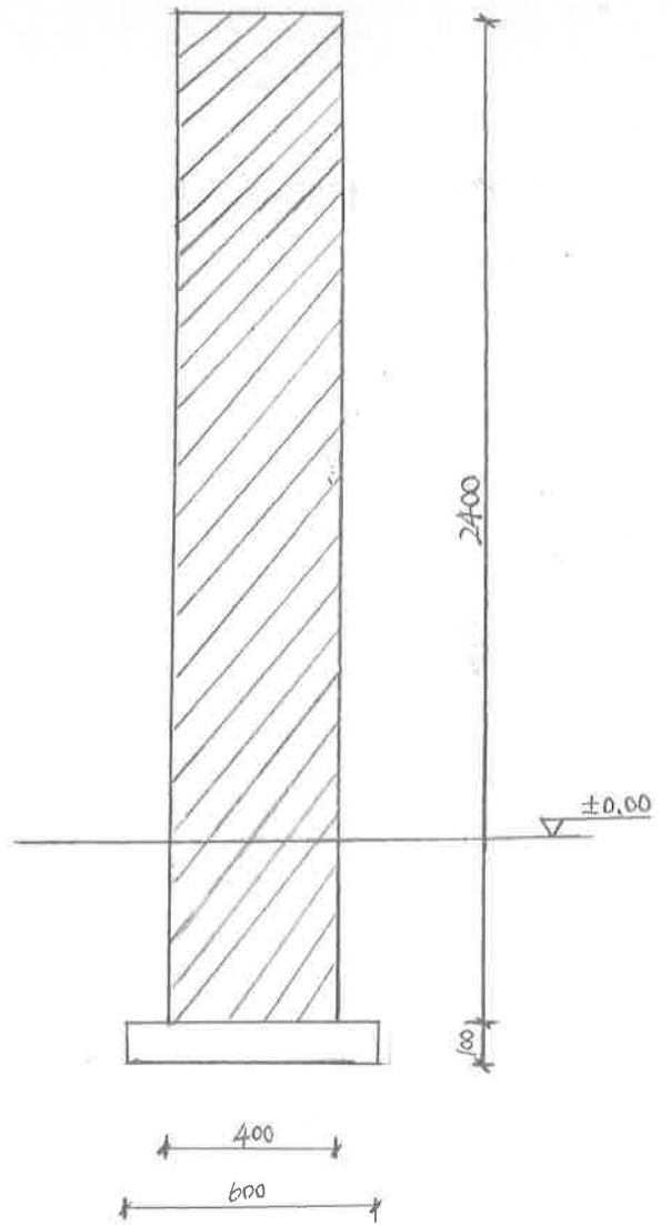
柱剖面 1:20
